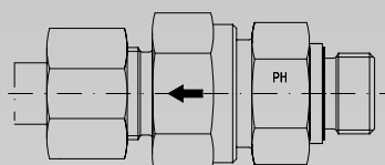
RV Strömung vom Einschraubzapfen Flow from Screwed Plug
