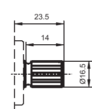
Tmax.=150 Nm 71 wielowypust B17x14 9 zębów; DIN5482
