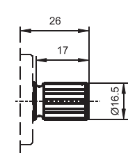
Tmax.=150 Nm 72 wielowypust B17x14 9 zębów; DIN5482
