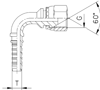
Końcówka 90°
