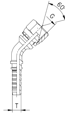
Końcówka 45°
