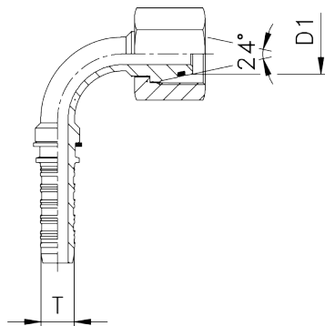
Końcówka 90°
