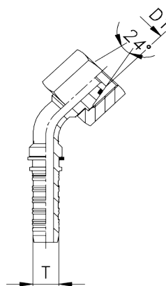
Końcówka 45°
